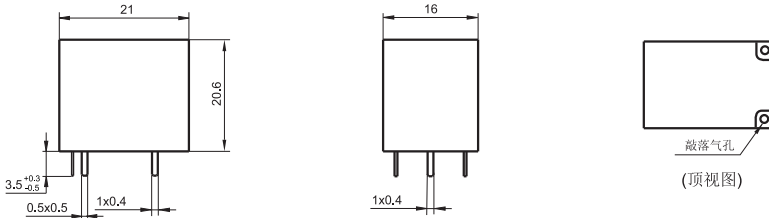
安装孔尺寸(底视图)
